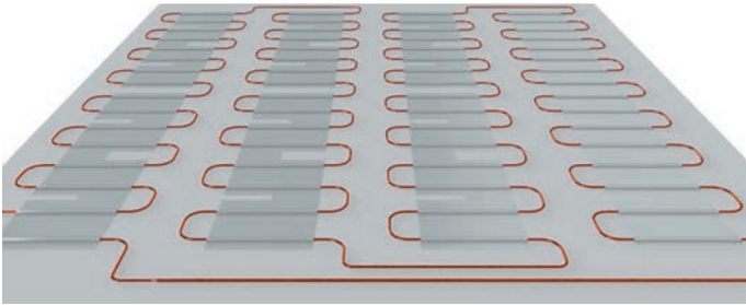
Normal-Kreis bis 15 m cufix ® ca. 1500 W; Abdecken mit PE-Folie 0,2
