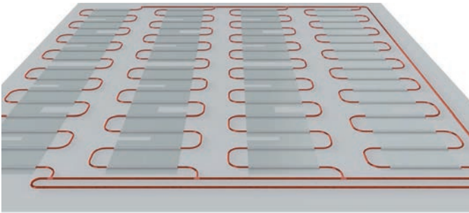
Tichelmann-Kreis bis ca. 8000 W; Abdecken mit PE-Folie 0,2
